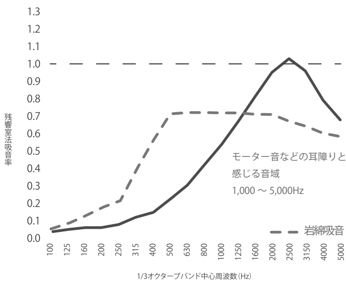
グラスウール 45K10T タイプ / 背後空気層：0mm
