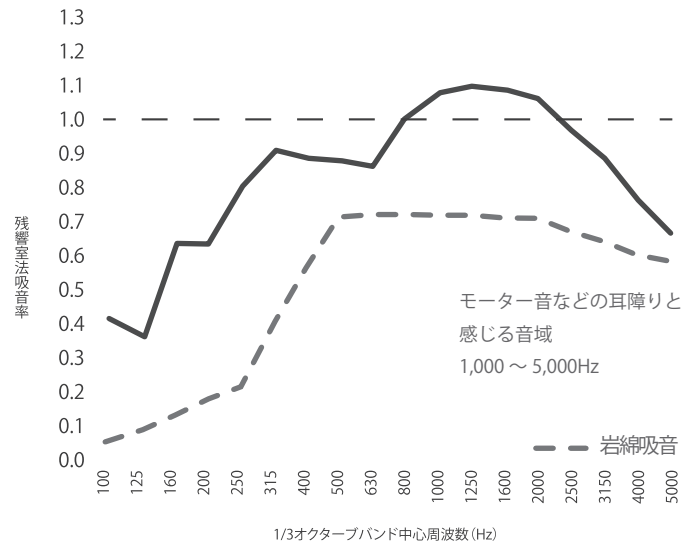
グラスウール 96K25T タイプ / 背後空気層：300mm
