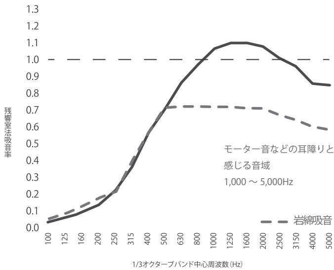
グラスウール 96K25T タイプ / 背後空気層：0mm
