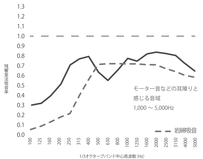
グラスウール 45K10T タイプ / 背後空気層：300mm
